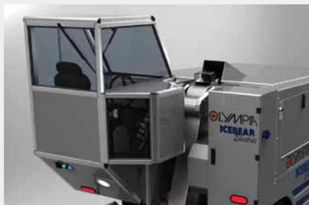
Hytt. Värmeutrustad hytt med mycket god sikt både framåt och bakåt. Utrustad med vindrutetorkare
